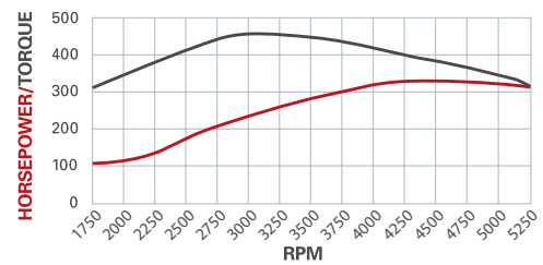
DYNO CHART
