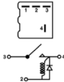
RY78 Cruise Control Relay E7TZ-13853A; E7TB 13853 A3B; E7SZ-13A025B; E6TZ-13853A; F8PZ 14N135 EA; F8PJ 14N135 EA; E6TA 13853 A; E6FZ-13853A; E6FZ-13853B; E6DZ-13853A; E9TZ-13853A; E9TB 13853 AA; E5EB-13853-B3A; E5EB-13853-B2A; E5EB-13853-B1A; E5EB-13853-A3A; E5EB-13853-A1A; E5EB-13853-A2A; E5DB-13853-A1A; D4DZ 13853 B; E4DB-13853-B1A; E4DZ-13853-B; E4DA-13853B; 12336289; 88922684
