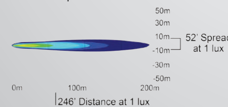
DURA-410 | 9891132 - 10° BEAM
