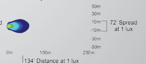
DURA-460 | 9141527 - 60° BEAM
