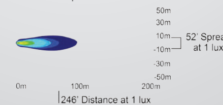
DURA-440 | 9141619 - 40° Beam
