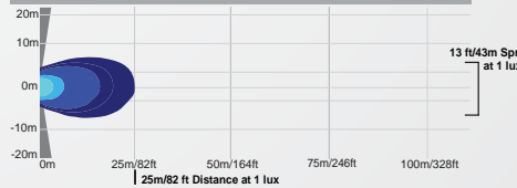
XIL-MX160 | 9113807 - 60° BEAM
