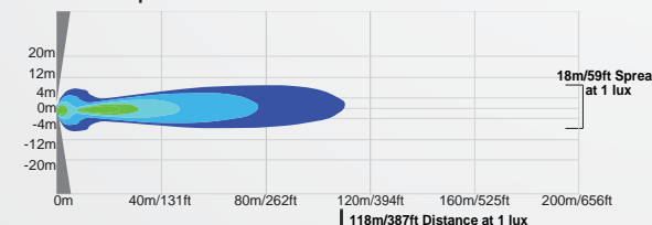
DURA-410 | 9891132 - 10° Beam
